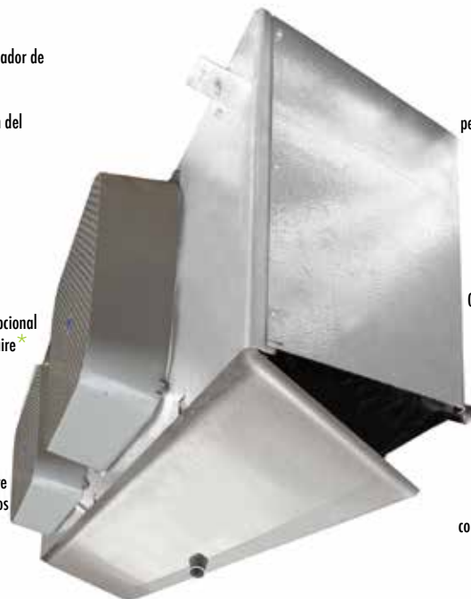
Diseño innovador del serpentín Thermo-Flex™ (patente U.S. No. 5,584,340) que elimina la posibilidad de fugas de refrigerante en los tubos que pasan por las cabeceras o secciones de soporte
