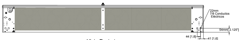
Vista Posterior
