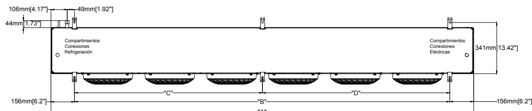
Vista Superior
